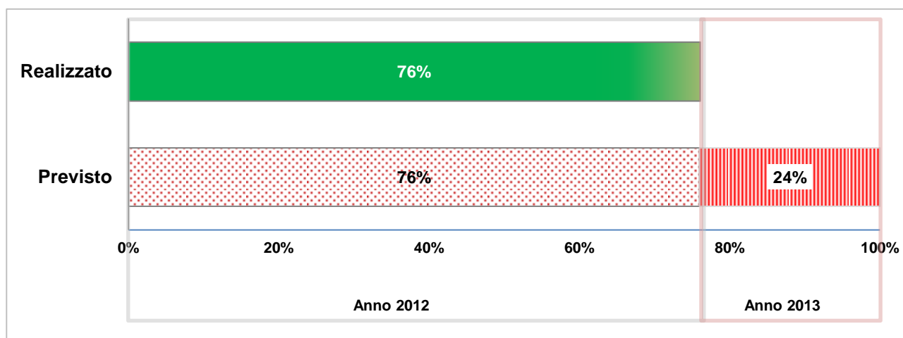
Figura 1.2.6.1: Confronto fra Stato Avanzamento Lavori (SAL) realizzato e previsto al 31 dicembre
