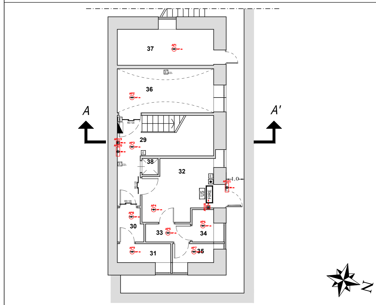
PROGETTO ESECUTIVO PIANO INTERRATO RILEVATORI scala 1:100
