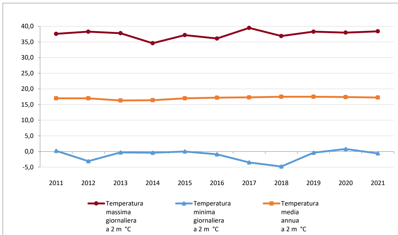
Graf.1.2 - Temperatura media, massima e minima giornaliera rilevate presso la stazione di Roma Via Lanciani. Anni 2011-2021
