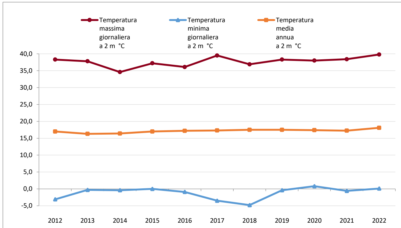
Graf.1.2 - Temperatura media, massima e minima giornaliera rilevate presso la stazione di Roma - Via Lanciani. Anni 2012-2022
