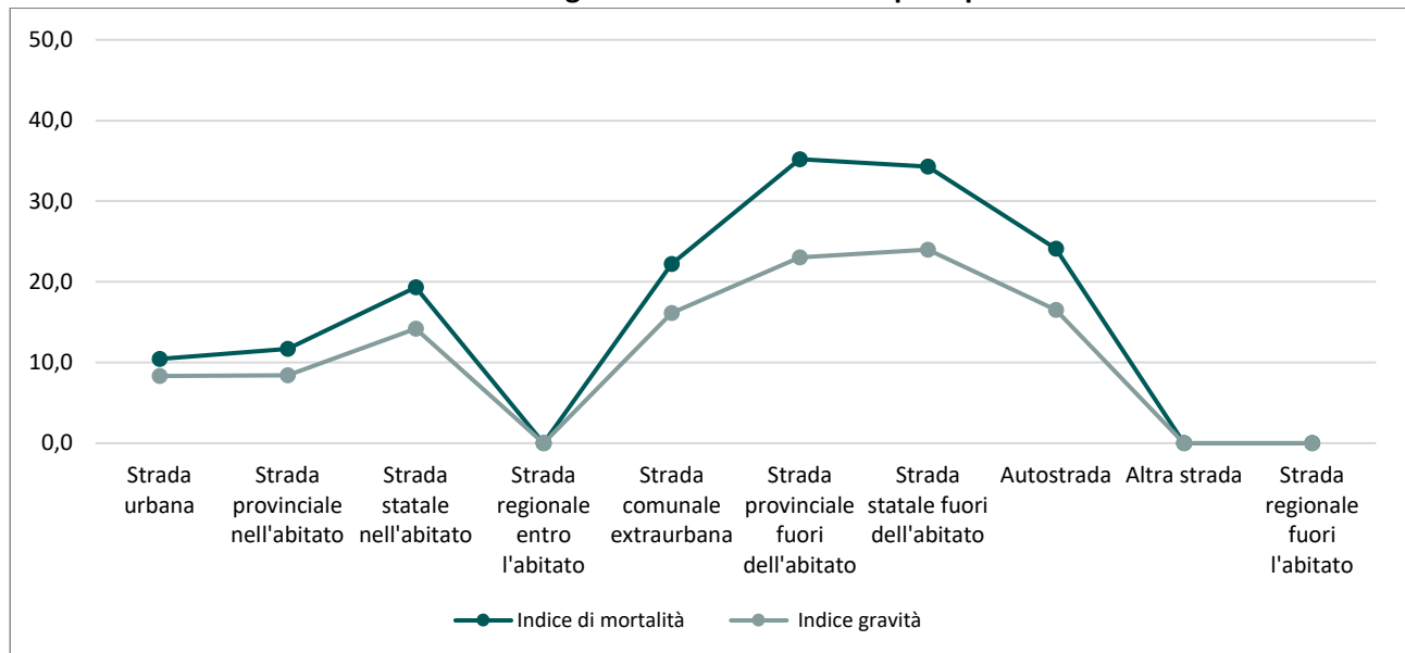
Graf.15.27 - Indice di mortalità e indice di gravità incidenti stradali per tipo di strada. Roma. Anno 2020
