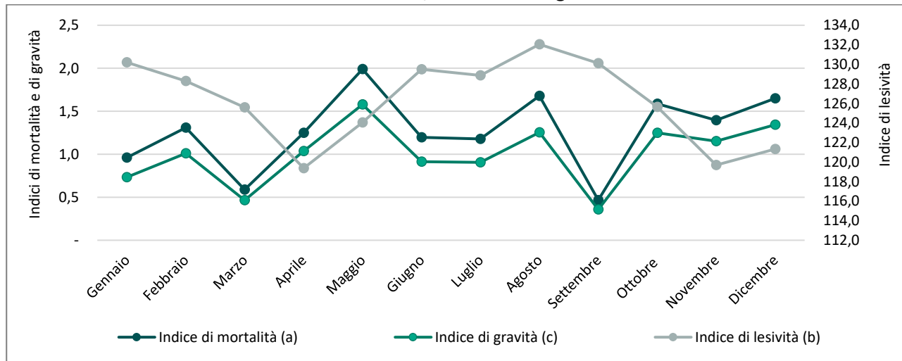
Graf.15.16 - Incidenti stradali: indice di mortalità, di lesività e di gravità. Roma. Anno 2020
