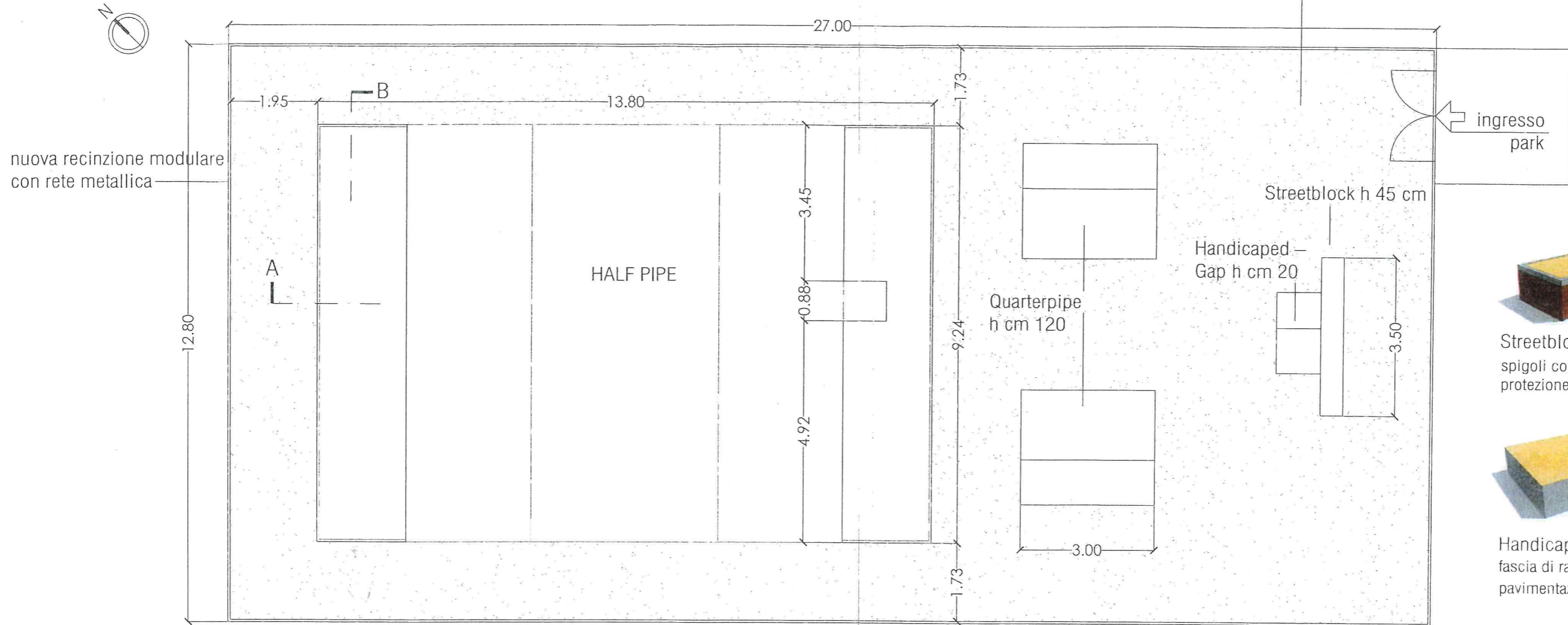
PLANIMETRIA rapp.: 1:100
