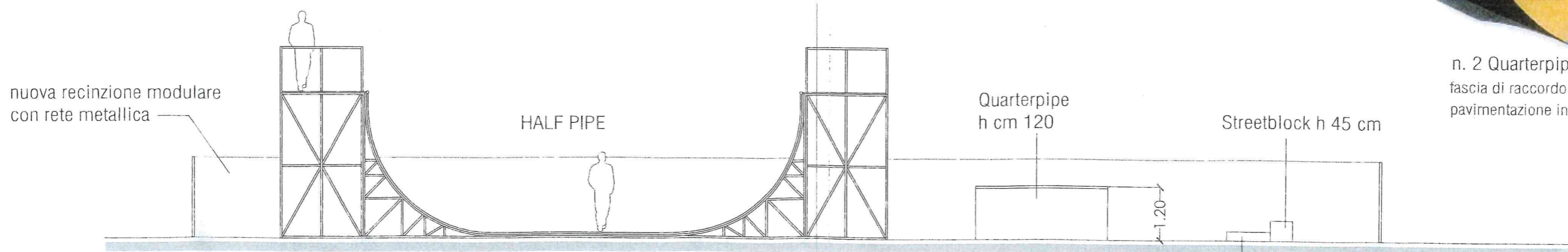
VISTA LATERALE rapp.: 1:100
