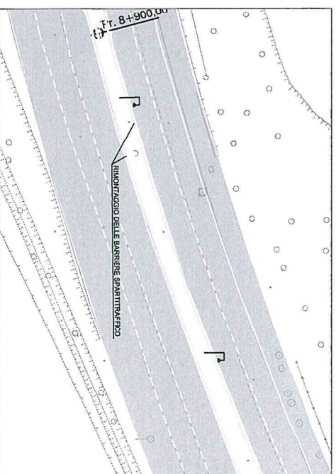
FASE 3: AL TERMINE DEI LAVORI SMONTAGGIO CUSPIDI E RIPRISTINO BARRIERE
