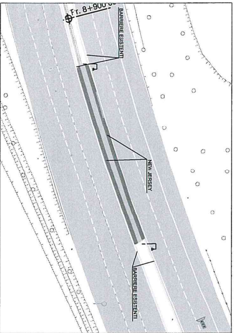
FASE 1: SMONTAGGIO BARRIERE E POSIZIONAMENTO NEW JERSEY PER LAVORI ALL'INTERNO DELLO SPARTITRAFFICO
